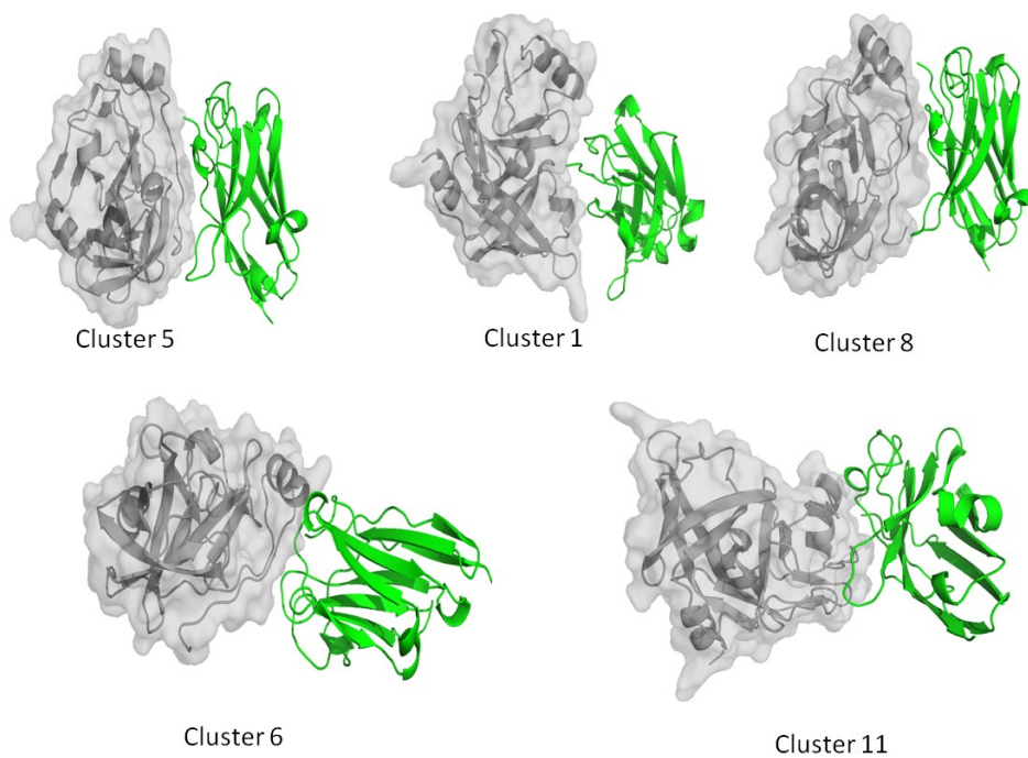
Clusters of NS3/4A-VH H 41
