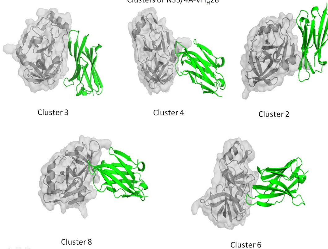
Clusters of NS3/4A-VH H 28
