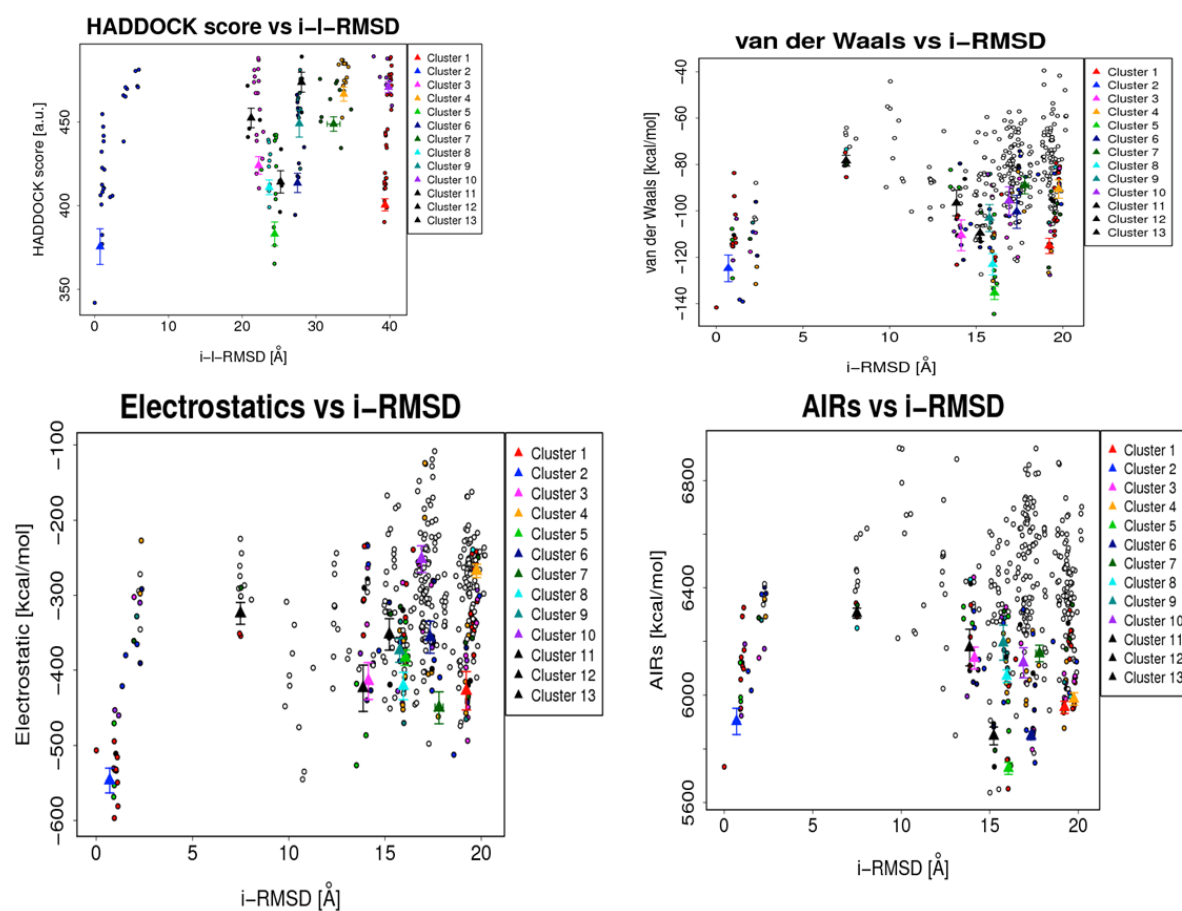
Clusters of NS3/4A-VH H 41
