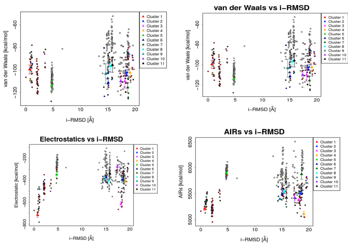
Clusters of NS3/4A-VH H 28
